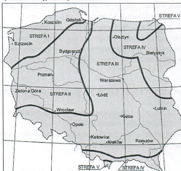
Rysunek 2. Strefy klimatyczne Polski.
